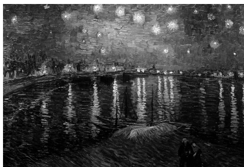
図1「ローヌ川の星月夜」
