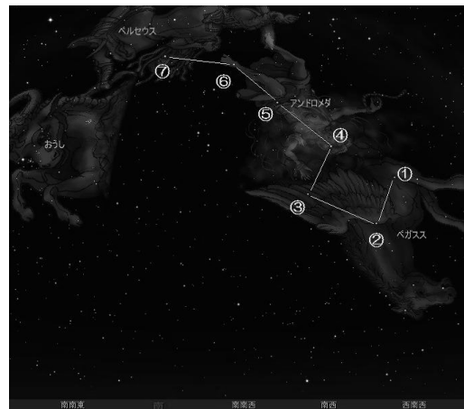
図6 「秋の大びしゃく」の星
