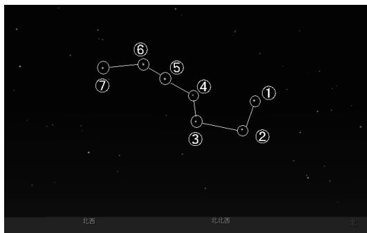
図4 北斗七星(ステラナビゲータで南仏アルルにおける1888年9月16日午後9時の北北西の空を再現し作図:以降の星図もすべてステラナビゲータで作図している)。北斗七星は常に北の空にあり、星②と①をつないで5倍のばすと北極星を見つけれられる。
