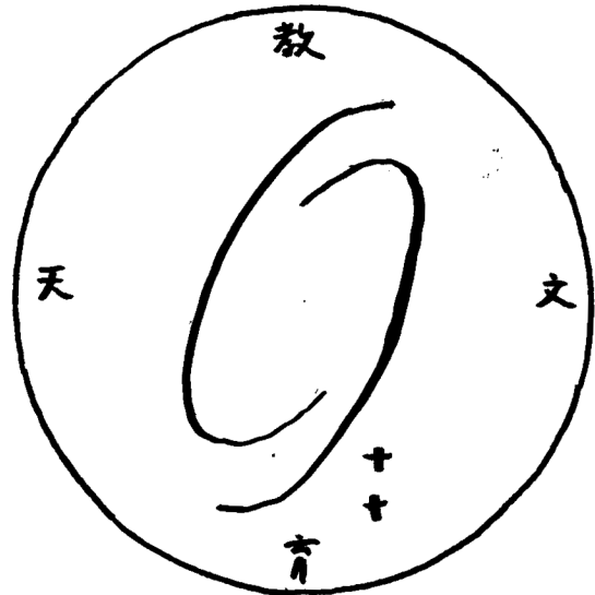
図 2 銀河
