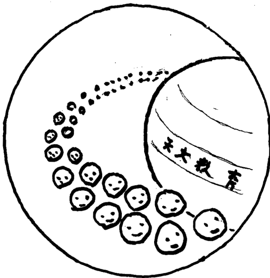
図 1 土星
